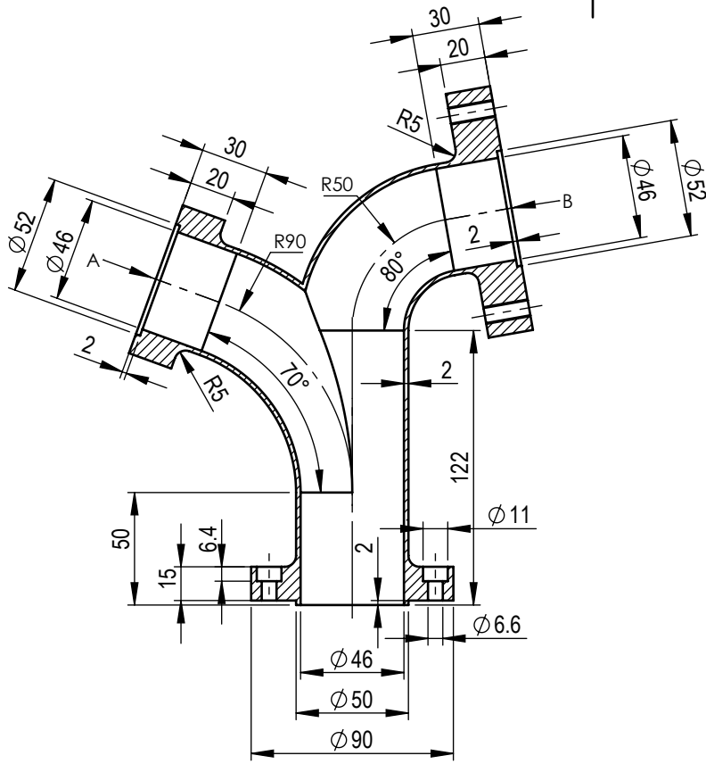
SECTION A-A SCALE 1 : 3
