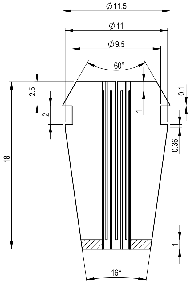
SECTION A-A SCALE 4 : 1
