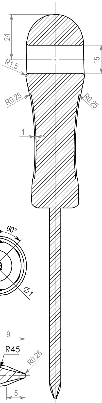
SECTION A-A SCALE 1 : 1
